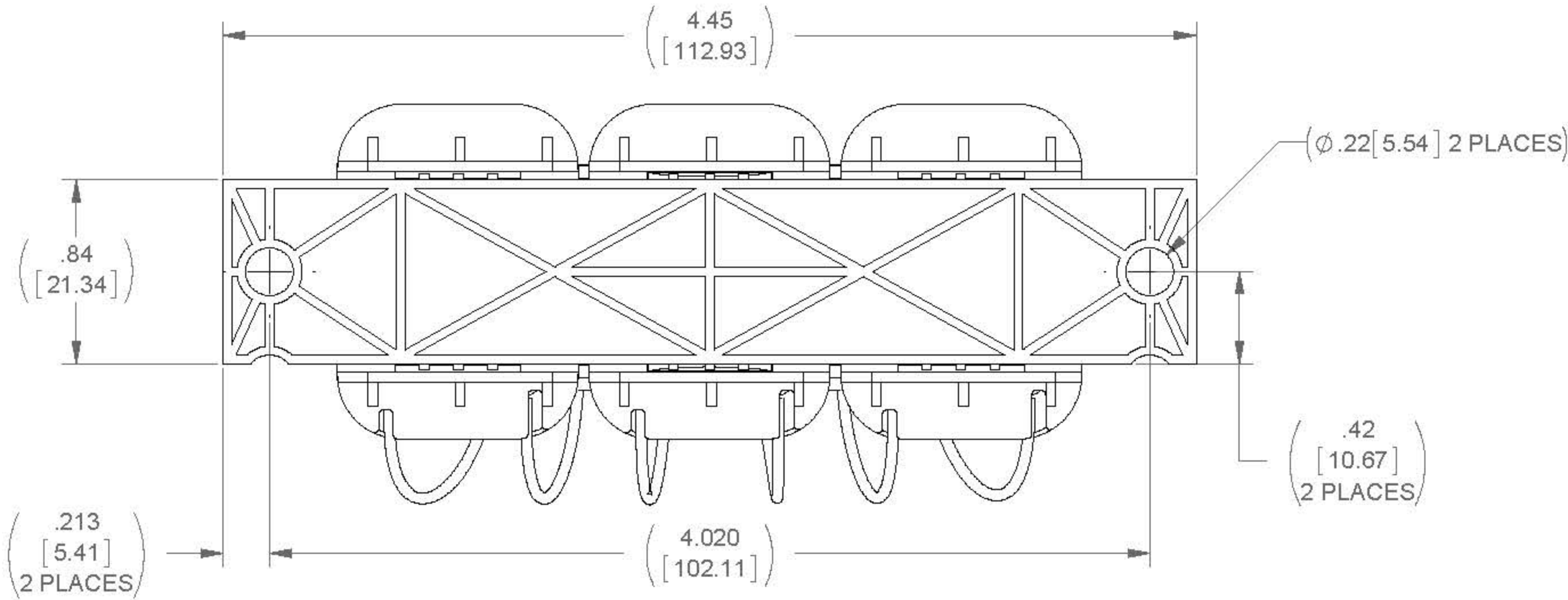
VIEW A-A
