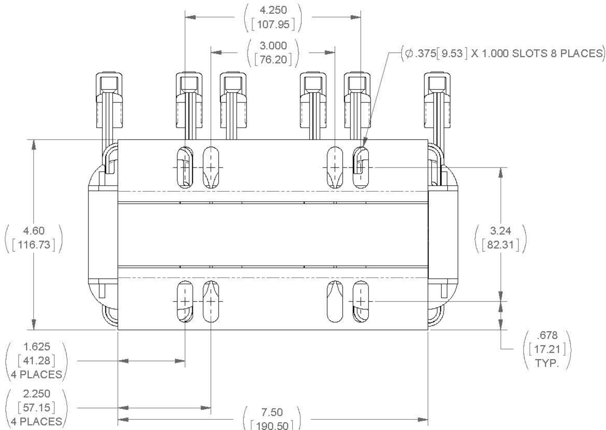
VIEW A-A
